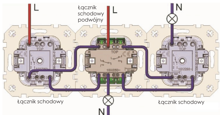
Układ podłączenia łącznika schodowego podwójnego z dwoma łącznikami schodowymi pojedynczymi.
