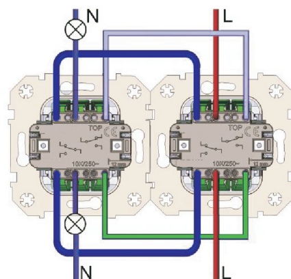
Układ podłączenia dwóch łączników schodowych podwójnych.
